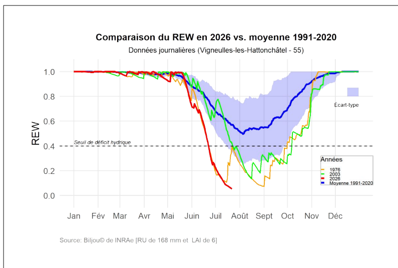
Modélisation de l'évolution de la réserve en eau disponible pour les arbres, réalisée à partir des données SAFRAN sur la maille de Vigneulles-lès-Hattonchâtel (55). Calculée avec l'outil Biljou© de INRAE (RU de 168 mm et LAI de 6).
