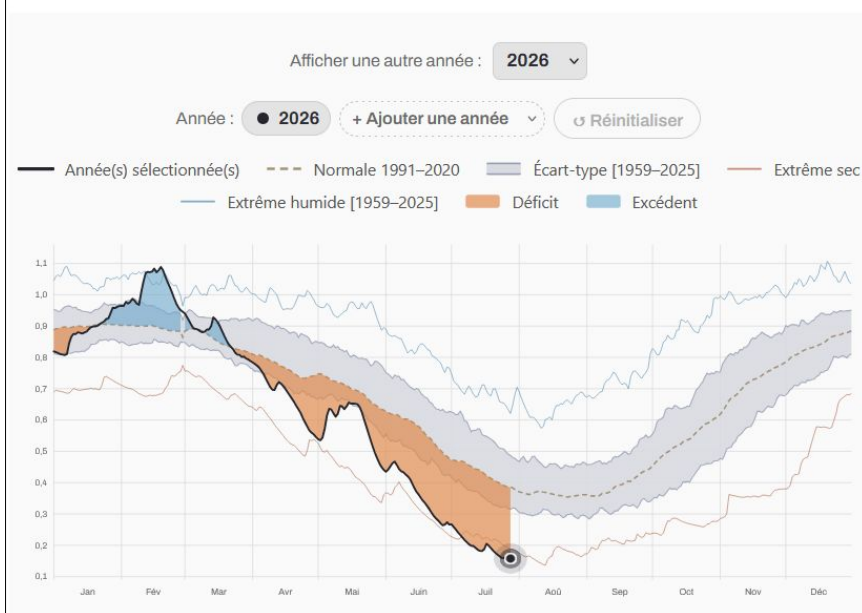
Indice d'humidité des sols superficiels sur la France du 1 er janvier au 28 juillet 2026 (© Météo-France)
